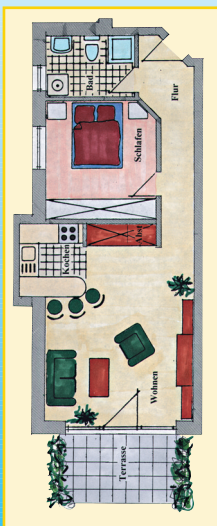
Grundriss der Wohnung
